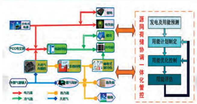
天府机场智慧能源管理系统
